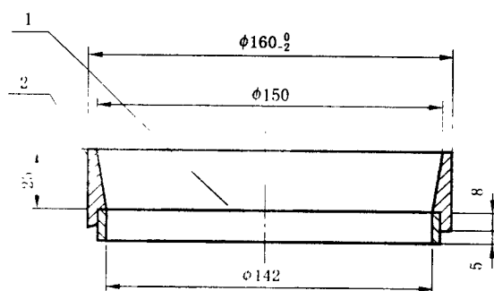
图 A.1 45 \mu\text{m} 方孔筛示意图
